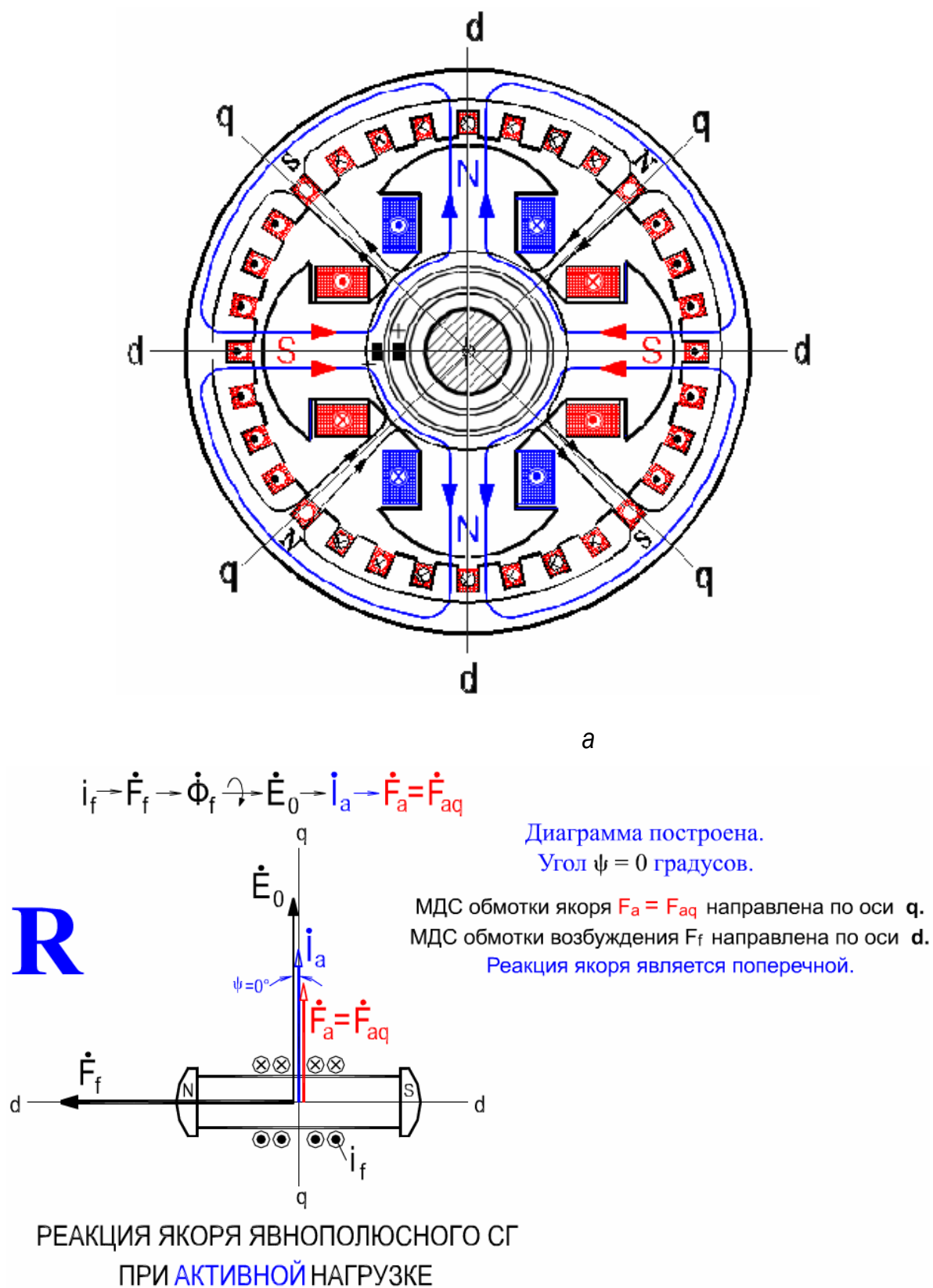
Рис. 7. Мультимедийные фрагменты видеолекции «Реакция якоря синхронной машины», иллюстрирующие в динамике влияние активной нагрузки, подключенной к обмотке якоря: а – взаимная ориентация магнитных полей якоря и индуктора; б – векторная диаграмма
